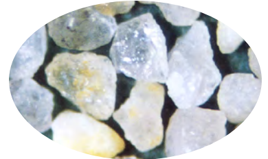
45メッシュサイズ顕微鏡写真 (拡大倍率30倍)
